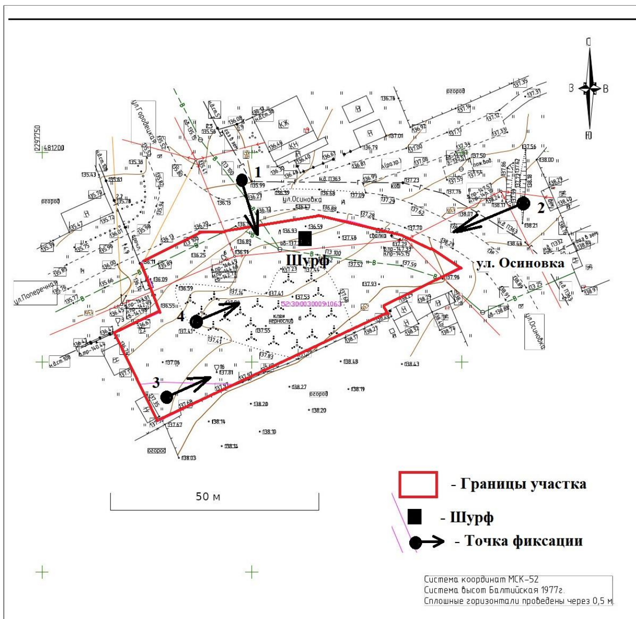
Ил.8. Нижегородская обл., Княгининский р-н, Ананьевский с/с, с. Егорьевское, ул. Осиновка, в 5 м на северо-запад от д. № 2. Топографическая схема участка обследования (предоставлена Заказчиком).
